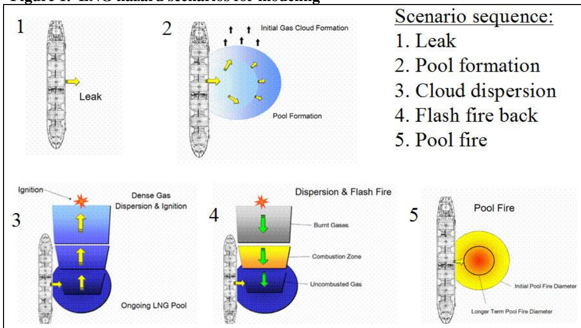
Figure 1. LNG hazard scenarios for modeling
